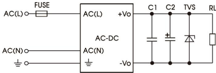
图 1: 典型应用电路
