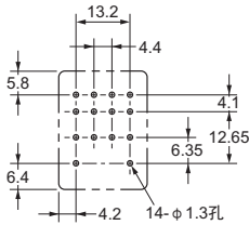
印刷电路板加工尺寸
