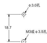
安装孔加工尺寸 (顶视图)
