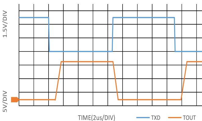
图6. 120kbps 的数据传输 (V CC =3.3V, R L =3kΩ)
