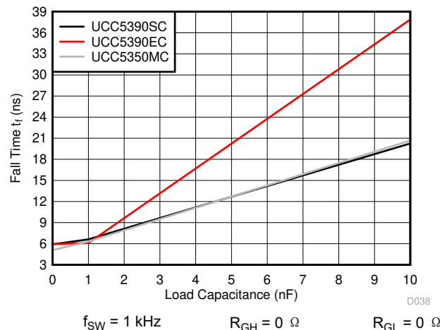
图 6-40. Fall Time vs Load Capacitance
